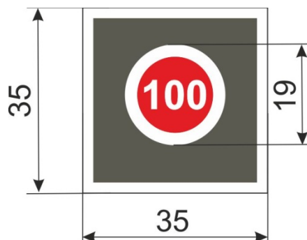
Рисунок 1 – Шеврон с указанием ЗЭТВ размером 35×35 мм
